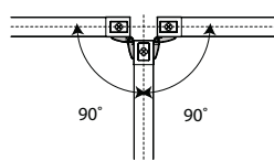
three-way junction connexion à 3 voies 3er Verbindung
